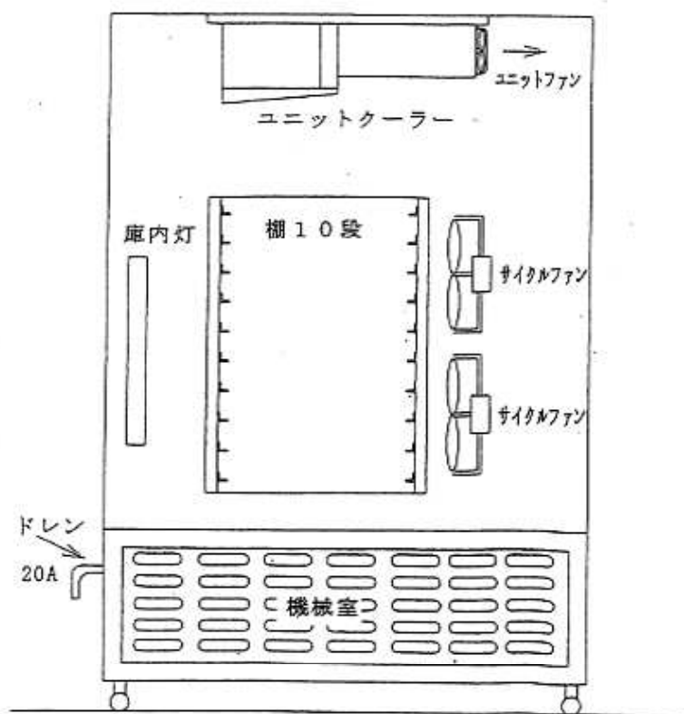
正面図
