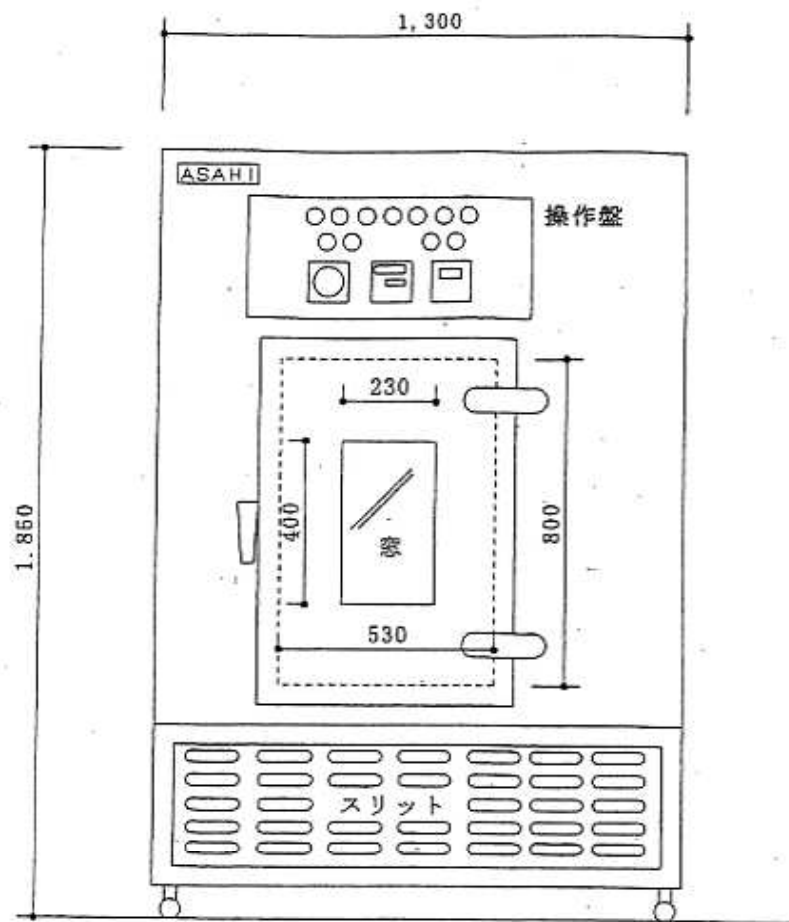
正面図
