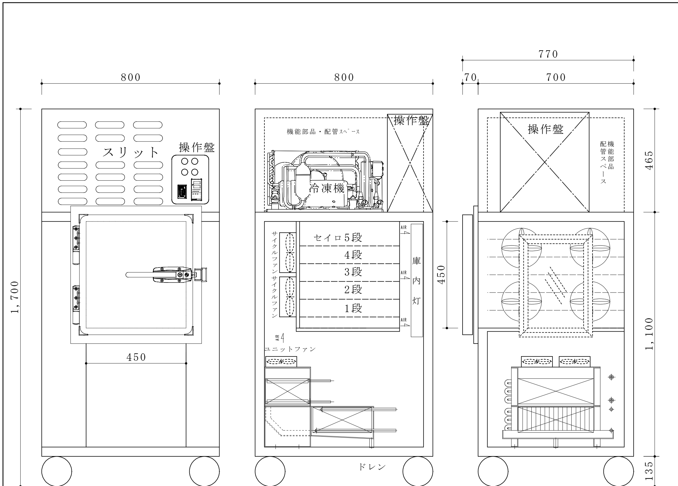
正面姿図
